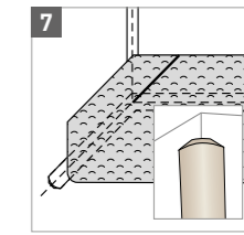
H204 Rohový profil CA12 pro stěnové fabion
