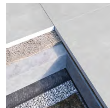
POKLÁDKA NA TERASE ALEBO PRÍJAZDOVEJ CESTE SLABO PRIEPUSTNÝ SUBSTRÁT
