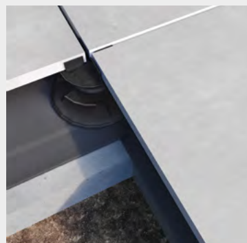
VYVÝŠENÁ POKLÁDKA NA PLOCHOM POKRYTÍ VYVÝŠENÁ PODLAHA NA TERASÁCH ALEBO BALKÓNOCH
