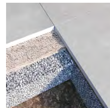
POKLÁDKA NA TERASE ALEBO PRÍJAZDOVEJ CESTE PRIEPUSTNÝ SUBSTRÁT
