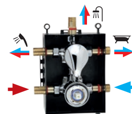
PŘÍKLAD ZAPOJENÍ box třícestný
